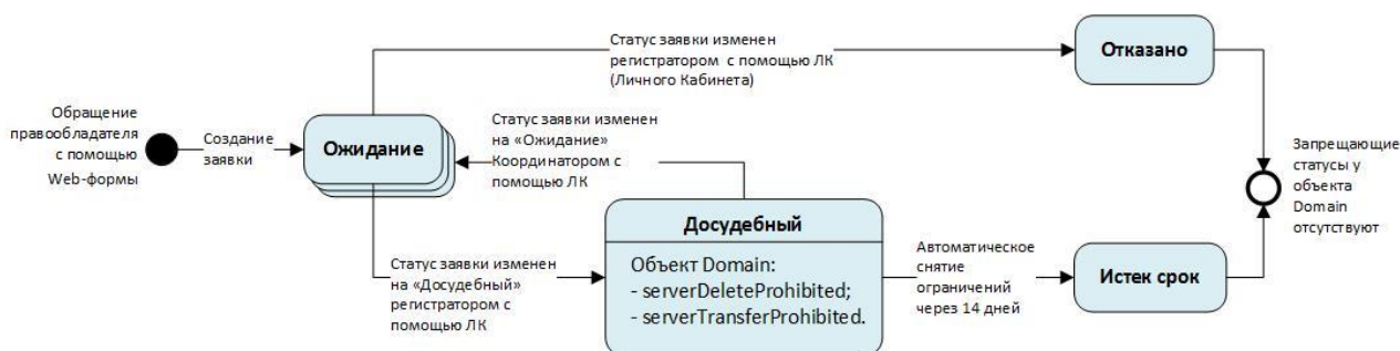
Рисунок 1. Жизненный цикл заявки
